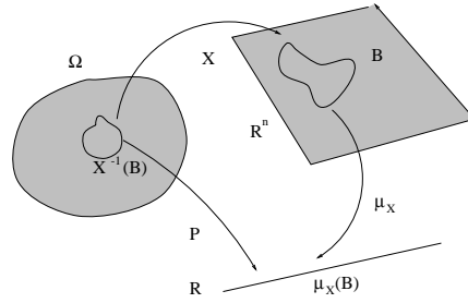
Σχήμα 1.1: Η κατασκευή του μέτρου \mu_X .
