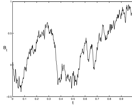
Σχήμα 3.1: Μία τροχιά της κίνησης Brown .
